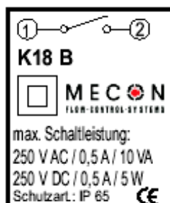
Fig. 8 Contact K 18 B
